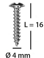
Schraube
