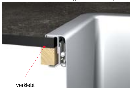
Abbildung 19: Befestigungsleisten verklebt
