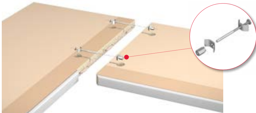
Abbildung 30: Arbeitsplatten-Verbinder
