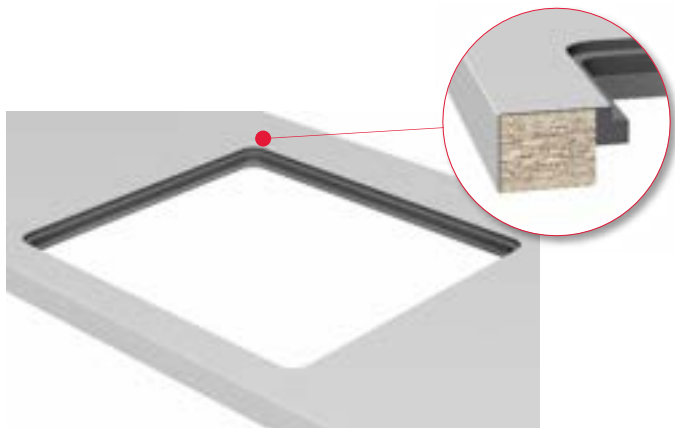
Abbildung 17: Flächenbündige Montage
